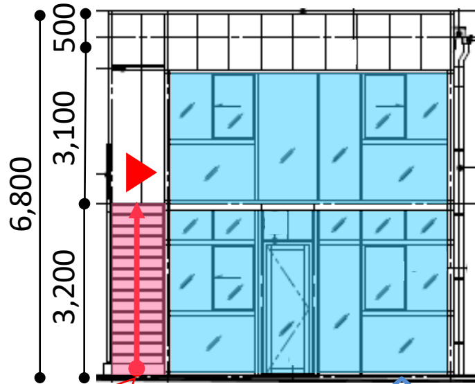
南立面図
