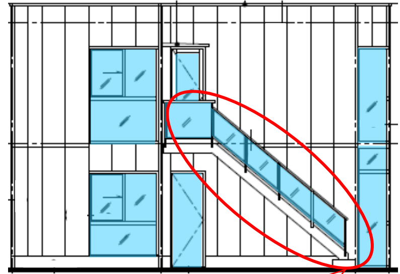
西立面図
